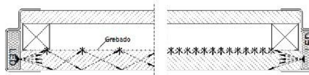
Diagrama esquemático
